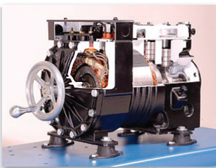
373-120 Semi-Hermetic Compressor
